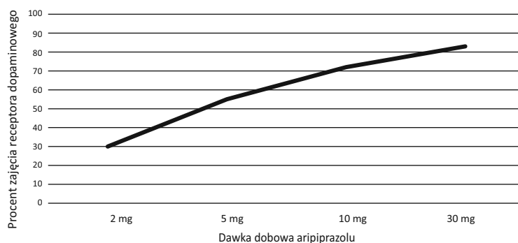
Rycina 2. Średnie zajęcie receptora dopaminowego D2 w zależności od dawki aripiprazolu
